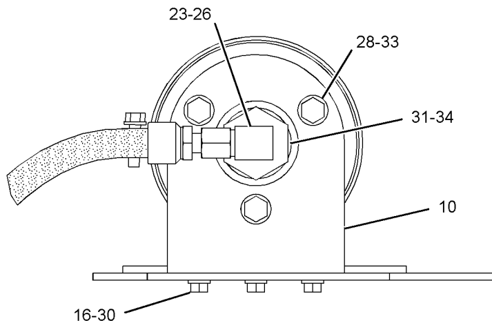
VIEW A-A
