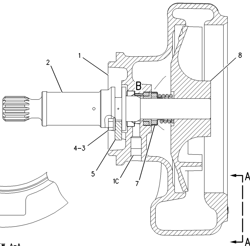
VIEW A-A
